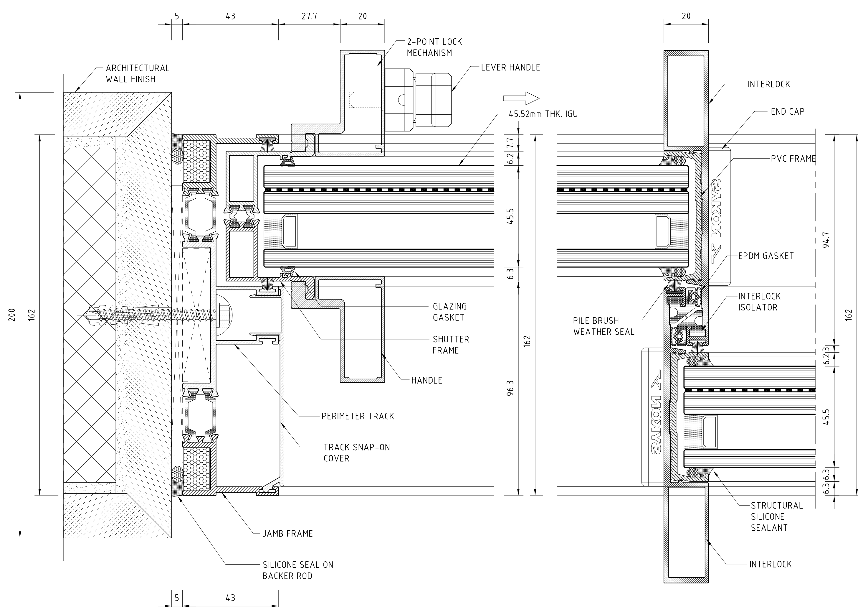
JAMB DETAIL
